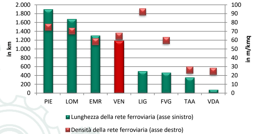
Rete ferroviaria (2014)
