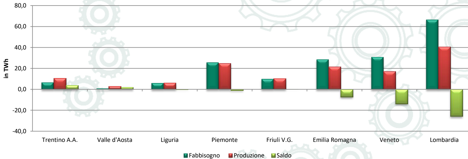
Bilancio elettrico (2016)
